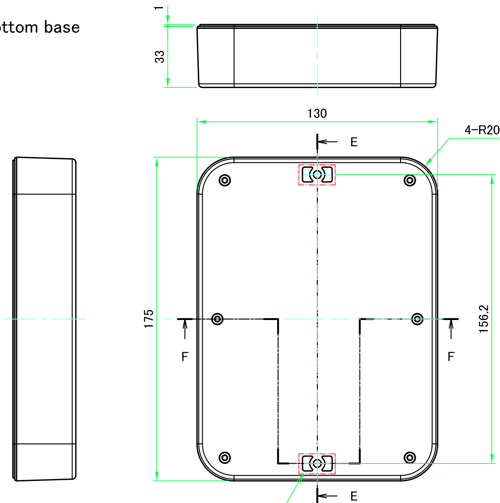
2-ポールマウントブラケット(WPMB-M4)用取付ガイド 2-Mounting position for Pole Mounting Bracket (WPMB-M4)
